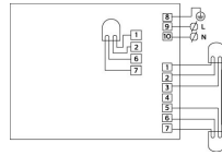
Scheda tecnica Philips HF-P 218 PL-T/C III 220-240V for 2x18W
